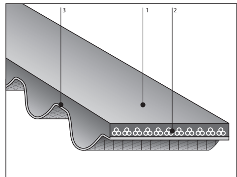
1.หน้ายางด้านหลัง 2.เส้นใยรับแรง 3.หน้าผ้าใบ
